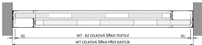
PŮDORYS - TYP AT-H-E
