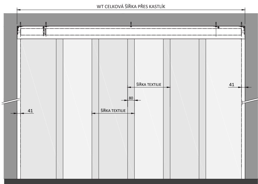
POHLED - TYP AT-H-E
