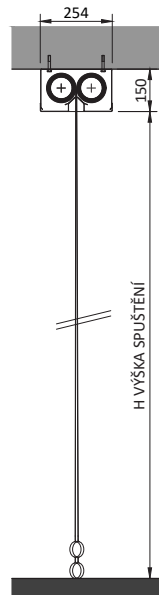
ŘEZ - TYP AT-H-E
